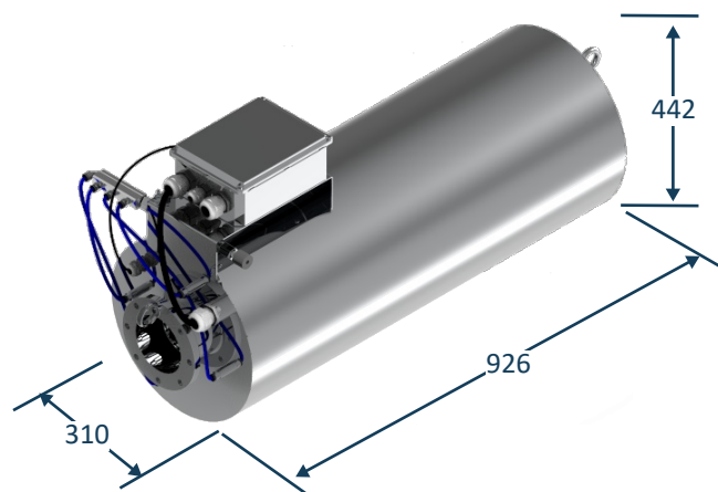
Medidas generador
